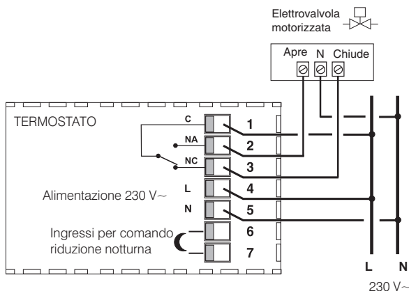
Fig. 4 - Esempio di collegamento a valvola motorizzata
