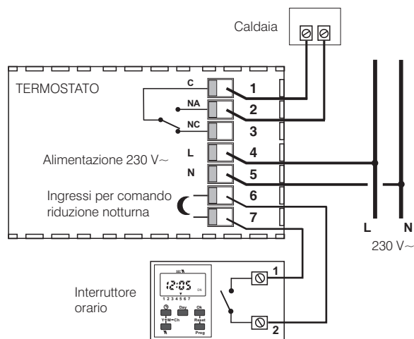
Fig. 3 - Esempio di collegamento a caldaia e orologio per comando riduzione notturna
